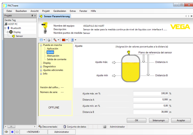
Fig. 11: Ejemplo de una vista de DTM - Configuración ajuste del sensor
