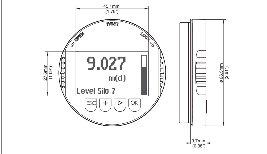
Fig. 12: Medidas módulo de visualización y configuración
